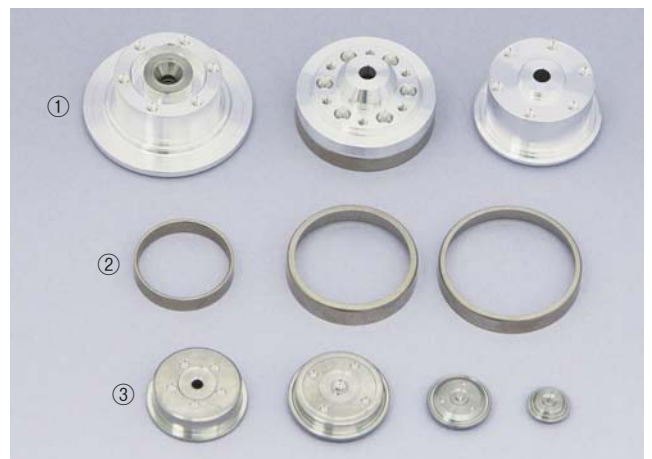
HDD用のハブ (①、③) と、ハブの付属部品ヨーク (②)
